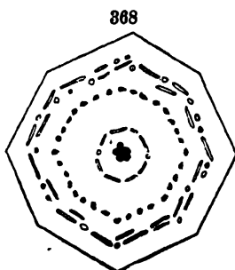
Leucite.
